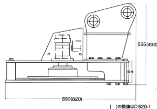
■ 寸法図
