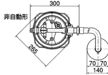
■外形寸法図 単位：mm
